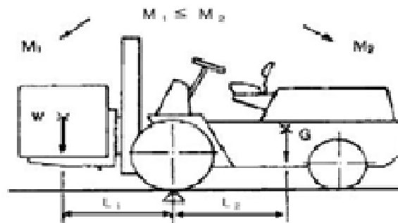
<그림 8> 지게차의 안정조건
