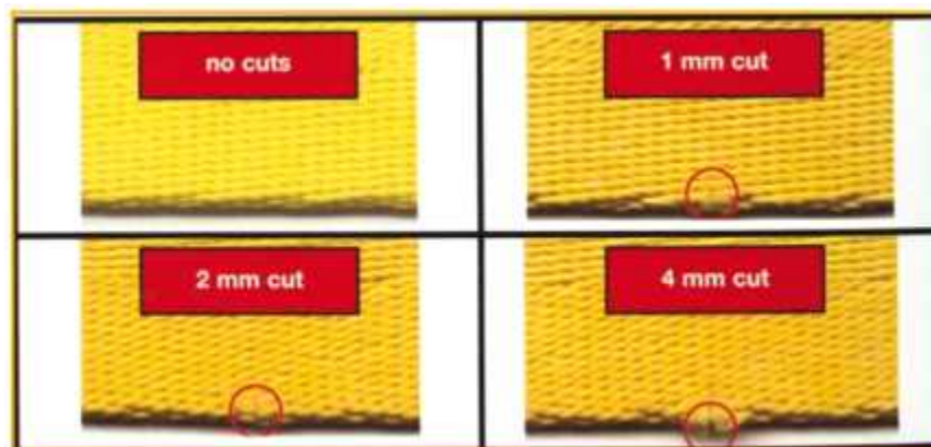
<그림 9> 웨빙 침줄의 절단 크기 비교 분석 (절단 크기가 강도 저하에 미치는 영향(1 mm 절단 시 5~40 % 강도 저하 가능성)을 시각적으로 보여줌)
