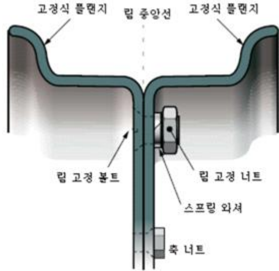
&lt;그림 8&gt; 분리형 휠의 교차 지점
