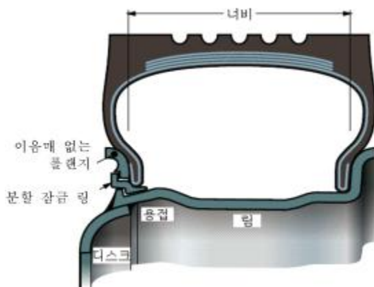
&lt;그림 5&gt; 3 피스 휠
