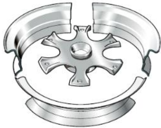
&lt;그림 6&gt; 분해 가능한 림
