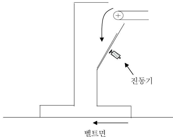
<그림 8> 슈트 경사면 진동기 설치
