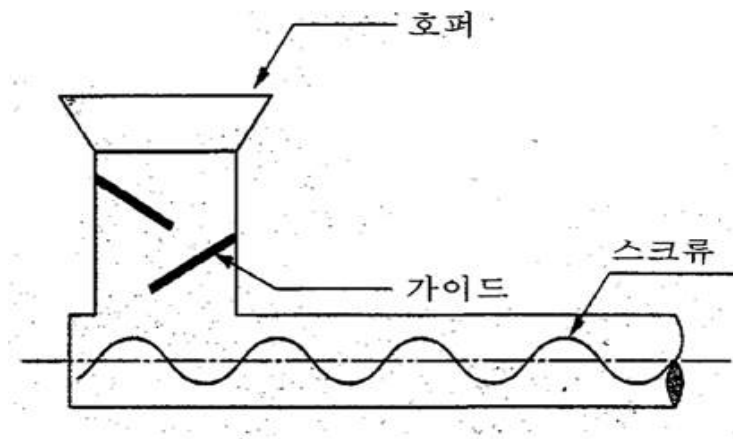
<그림 2> 내면가이드 설치도
