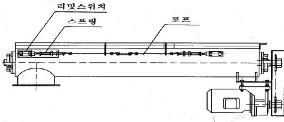
<그림 6> 잠금용 로프식 연동장치 설치도
