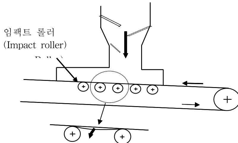
<그림 9> 벨트면과 스커트사이 틈 최소화를 위한 임팩트 롤러 간격 조정
