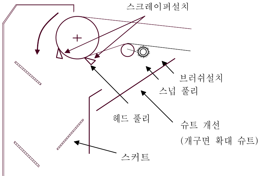
<그림 13> 헤드측의 안전조치
