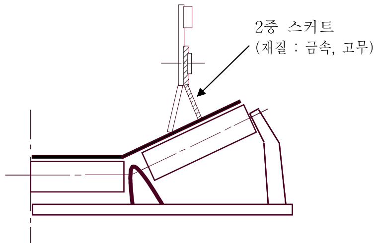
<그림 10> 2중 스커트
