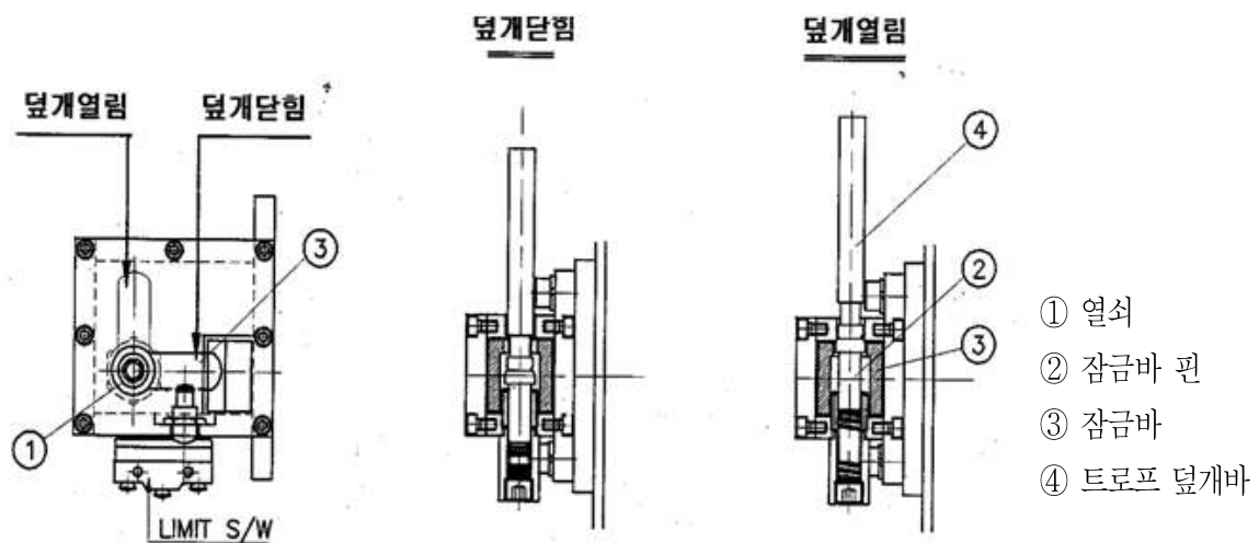
“잠금바 잠금장치” 상세도 “트로프 덮개바 잠금장치” 상세도
