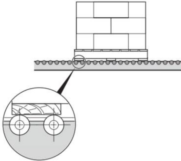
<그림 8> 팔레트 컨베이어의 롤러 간격은 바닥 지지대의 길이보다 짧아야 함
