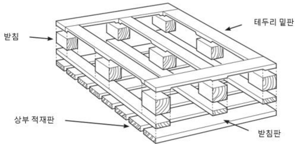
<그림 12 ㉞> 4방향 차입식 팔레트(아래쪽에서 본 모습)
