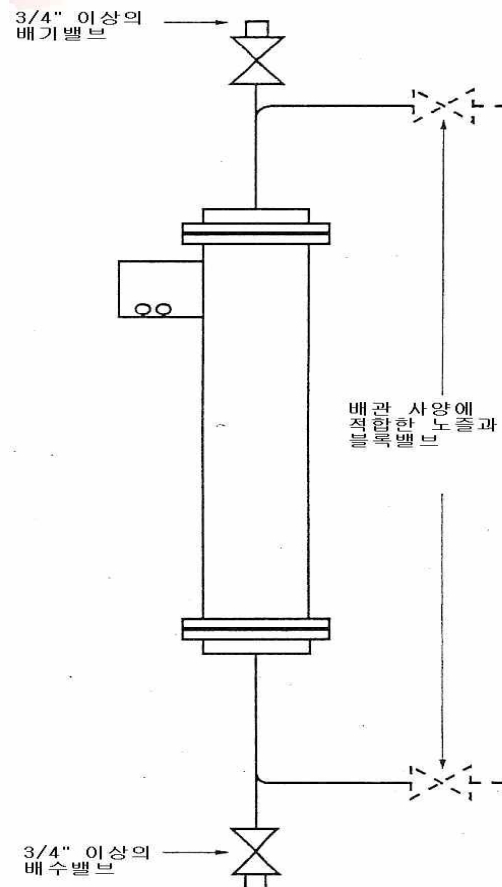
<그림 11> 외장 변위 전송기의 스탠드파이프
