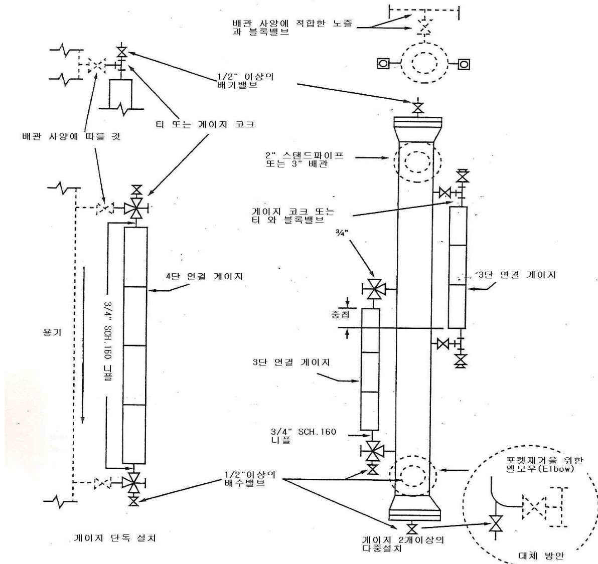
<그림 8> 게이지 설치
