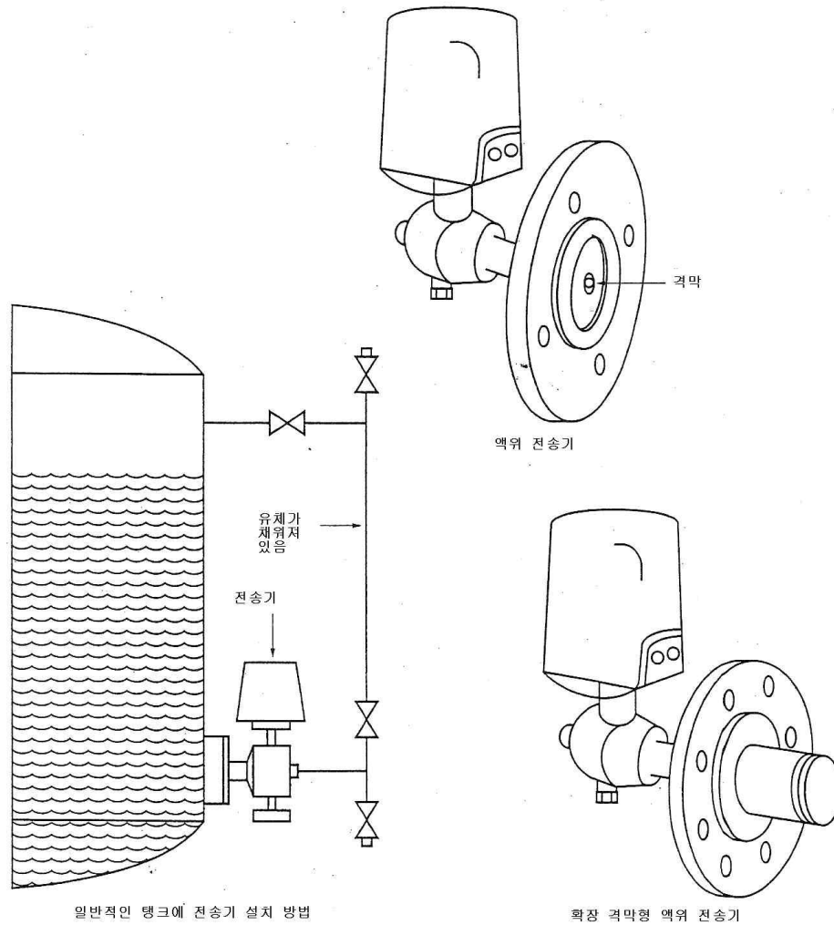
<그림 14> 플랜지 체결 차압 전송기의 설치
