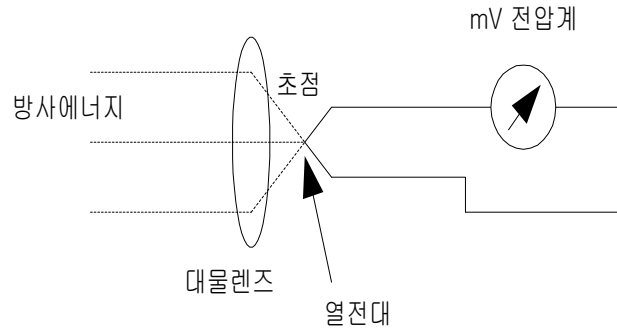
<그림 5> 방사식 온도계의 측온방법
