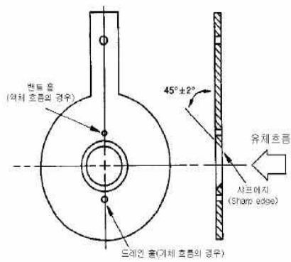
(a) 정중앙오리피스
