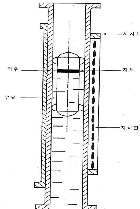
<그림 7> 자기 액위계
