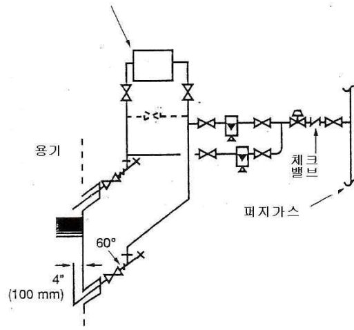
C-퍼지 가스를 사용한 차압식 액위 전송기
