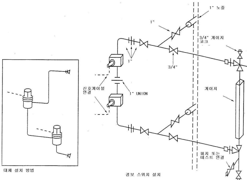
<그림 15> 게이지에 병렬로 경보 스위치 설치
