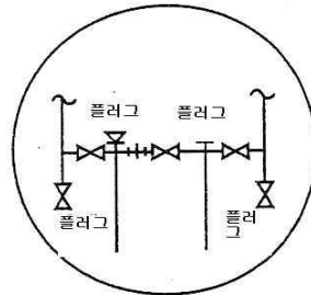
B-실링 (SEALING) 유체를 사용한 경우
