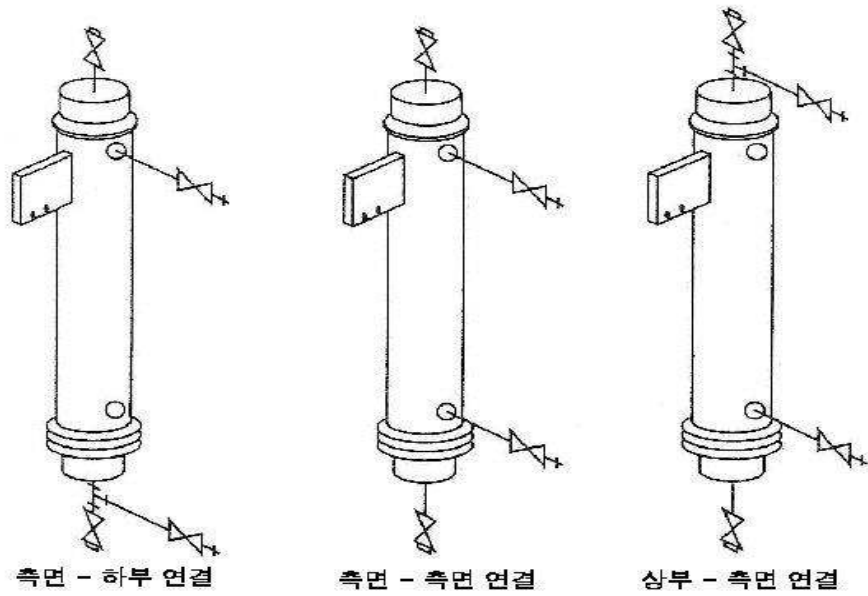
<그림 10> 외장 변위 전송기의 설치
