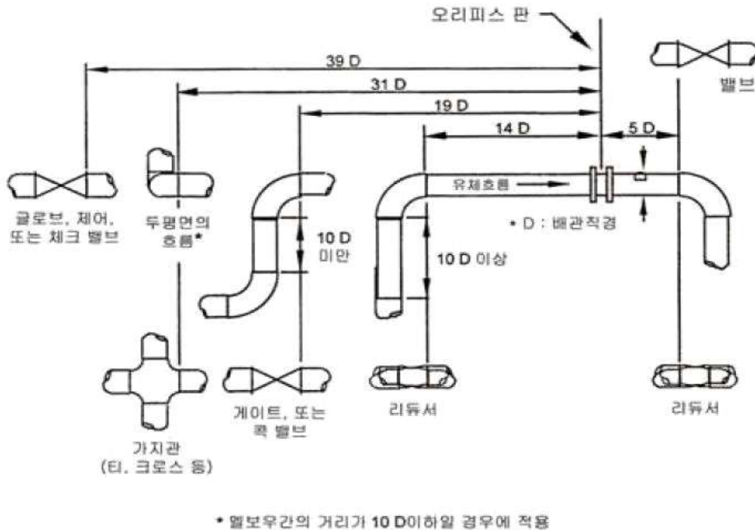
<그림 6> 오리피스 직관부에 요구되는 최소 거리 (AGA-ASME Fluid report #3에 근거)
