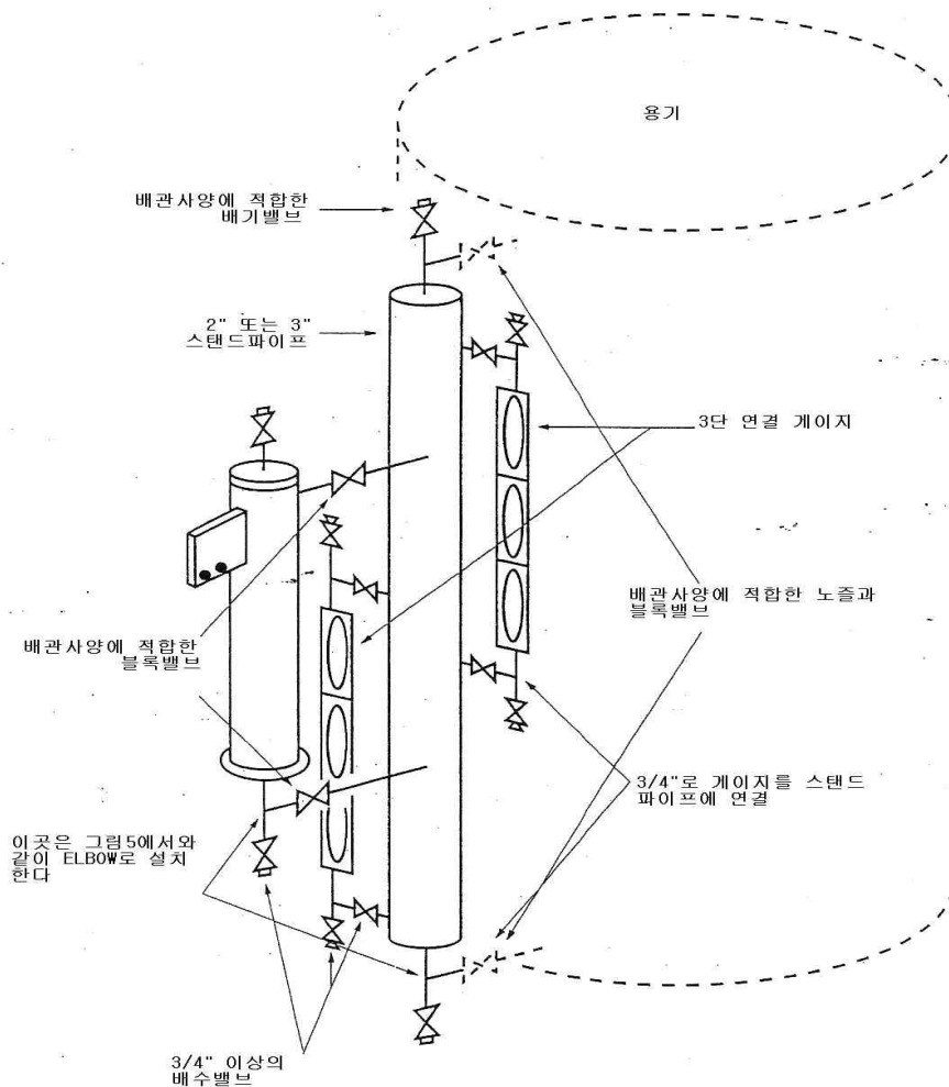
<그림 12> 외장 변위 전송기의 스탠드파이프를 이용한 다중설치
