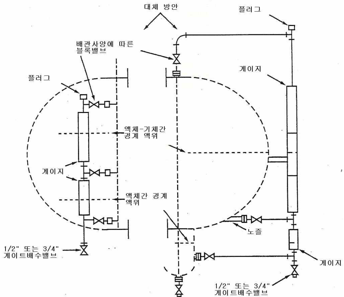
<그림 9> 경계 액위 측정을 위한 게이지 설치
