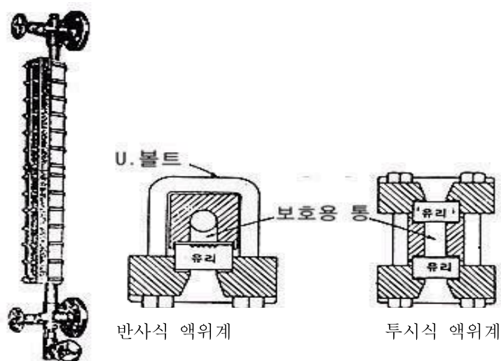
<그림 1> 외장 유리액위계
