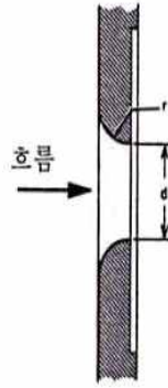
(b) 사분원오리피스
