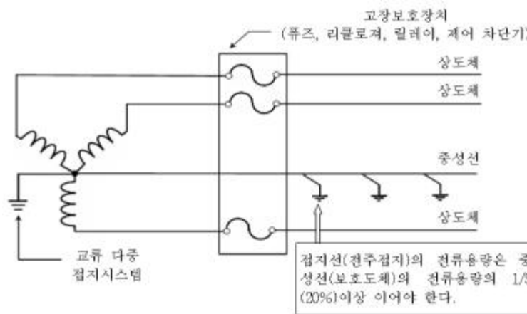
<그림 2-4> 교류 다중접지시스템에서의 접지선
