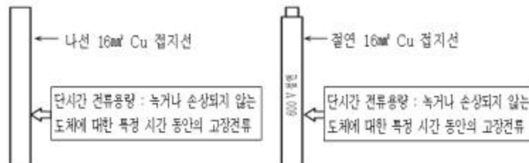
<그림 2-2> 절연 접지선과 나선 접지선의 단시간 전류용량
