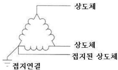
(c) 코너 접지된 3상3선식 △결선 회로
