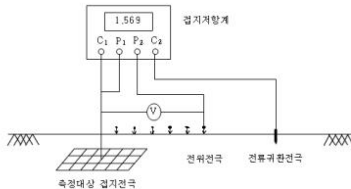
<그림 3-2> 대형 접지극의 접지저항 측정회로
