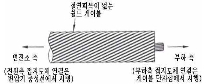
<그림 6> 절연피복이 없는 쉴드 케이블의 접지
