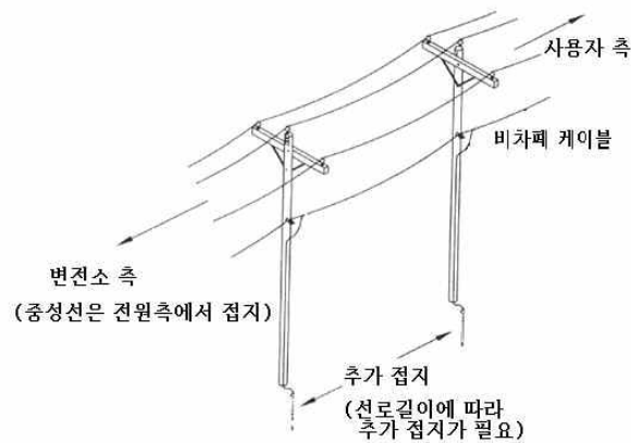
<그림 5> 600 V 이상의 가공선로에서 비차폐 케이블의 접지
