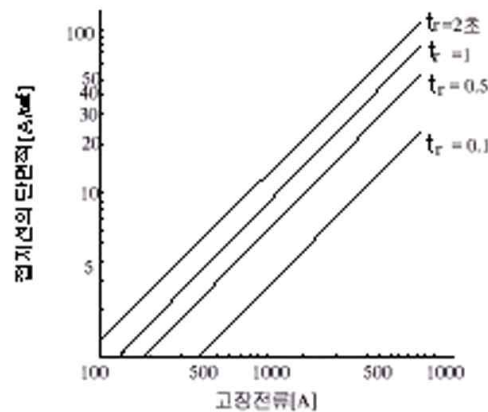
〈그림 2〉 고장전류와 접지선 굵기의 관계
