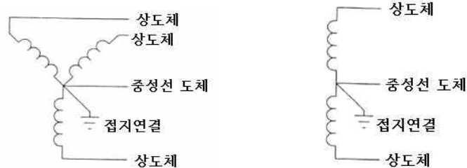
(a) Y 결선 3상4선식 교류계통 (b) 단상 3선식 교류계통 <그림 2> 저압 교류계통에서의 접지 연결지점
