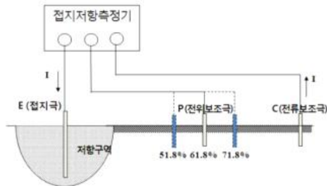
<그림 3-3> 허용폭을 이용한 접지저항 측정방법
