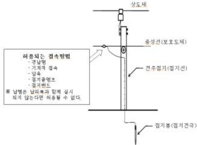
<그림2-1> 접지선과 보호도체의 접속
