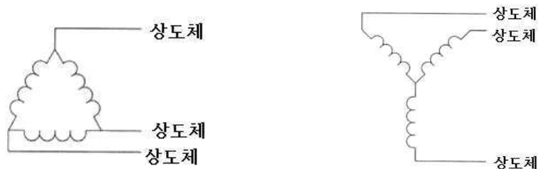
(a) 비접지 3상3선식 △결선 회로 (b) 비접지 3상3선식 Y결선 회로
