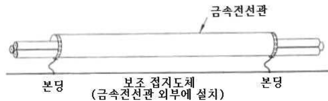
<그림 8> 본딩이 된 금속전선관
