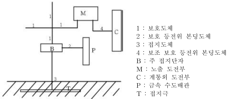
<그림 1> 접지선 및 접지도체의 예
