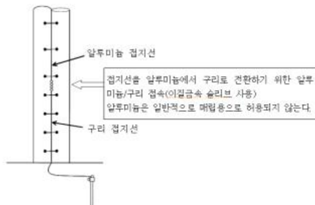
<그림 2-8> 매립용 구리로 전환하기 위한 알루미늄 접지선의 예
