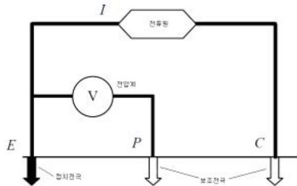
<그림 3-1> 소형 접지극의 접지저항 측정회로
