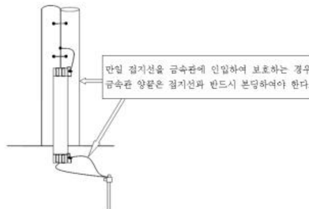
<그림 2-7> 금속관에 접지선을 인입하는 경우의 요구조건
