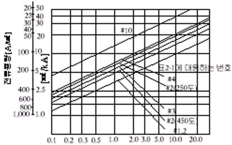
통전시간(초) <그림 1> 접지선의 전류용량
