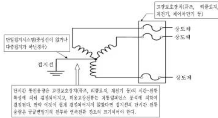
<그림 2-3> 단일접지시스템에서의 접지선
