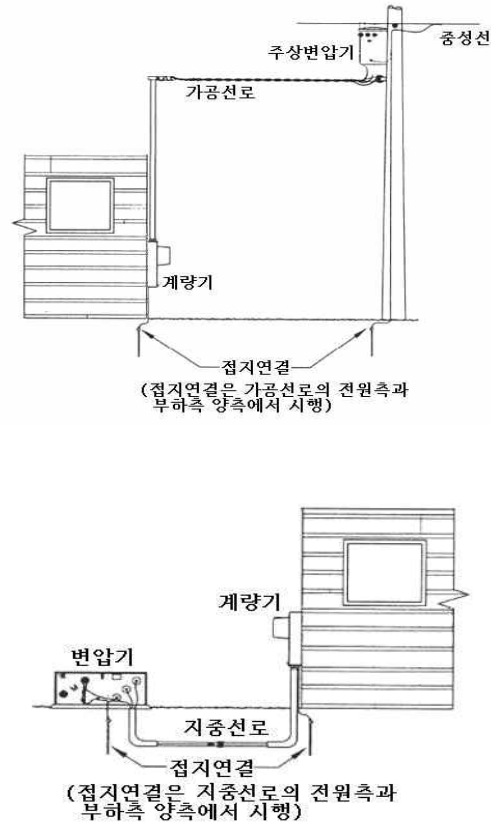
<그림 4> 저압 교류계통에서의 접지 연결지점
