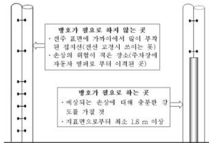
<그림 2-6> 방호의 유무에 따른 접지선에 대한 필요조건
