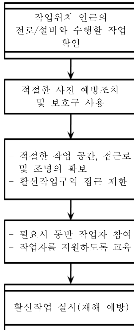
<그림 4> 활선작업에 대한 작업절차의 평가
