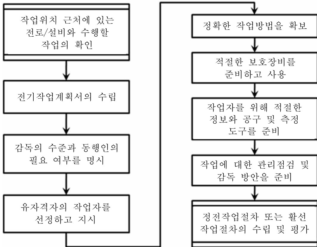
<그림 2> 정전 및 활선작업에 공통되는 조치의 평가
