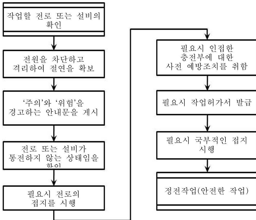
<그림 3> 정전작업에 대한 작업절차의 평가
