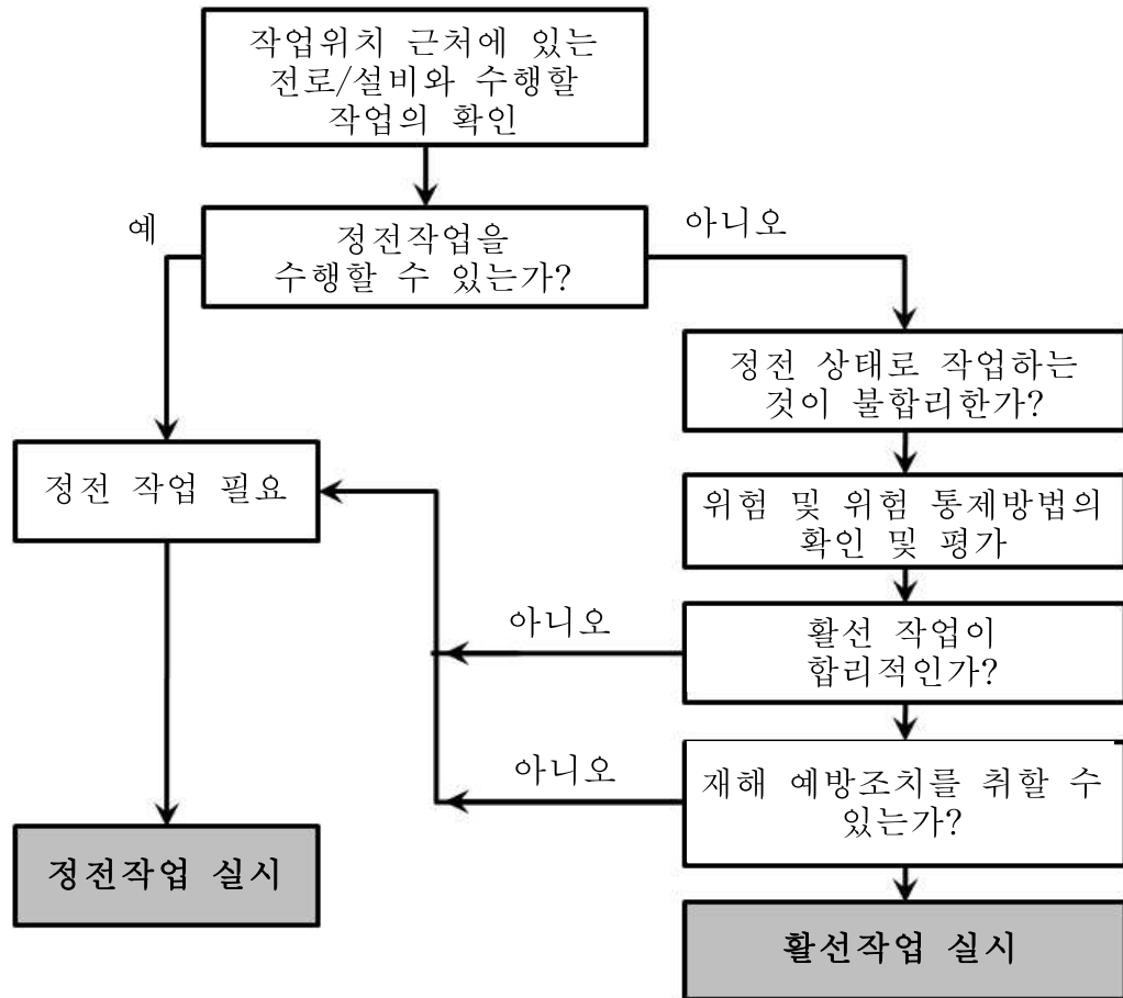
<그림 1> 정전작업 또는 활선작업 여부의 평가 및 판단
