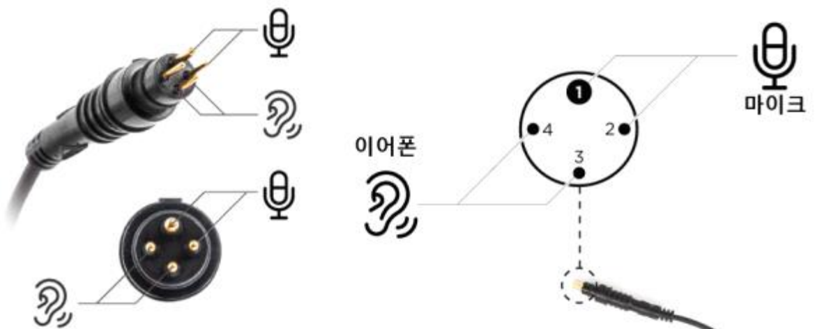
<그림 4> 잠수헬멧측 통화장치용 수(male) 방수 커넥터
