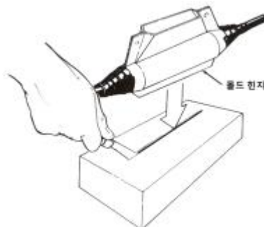
<그림 7> 몰드 세우기
