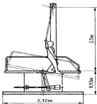
(그림 1) 경사로(ramp tester) 시험기 구조 및 사진
