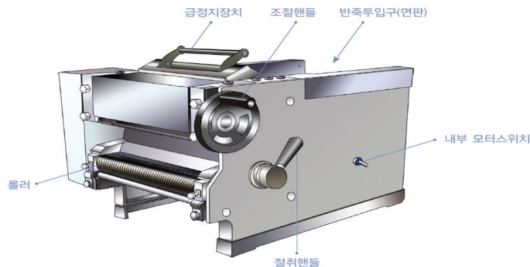
(그림 13) 제면기의 구조
