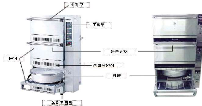
(그림 1) 가스 자동밥솥 구조
