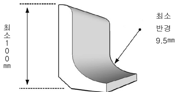
(그림 3) 벽체와 바닥의 이음매 부위(굽도리널)
