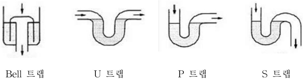
(그림 4) 트랩의 종류에 따른 형상(예)
