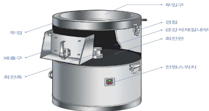
(그림 14) 감자탈피기의 구조
