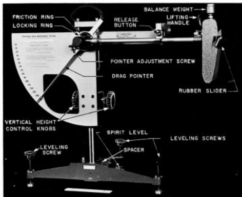
(그림 1) Pendulum Tester사진
