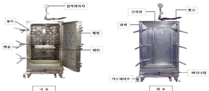
(그림 2) 다단 취사기 구조
