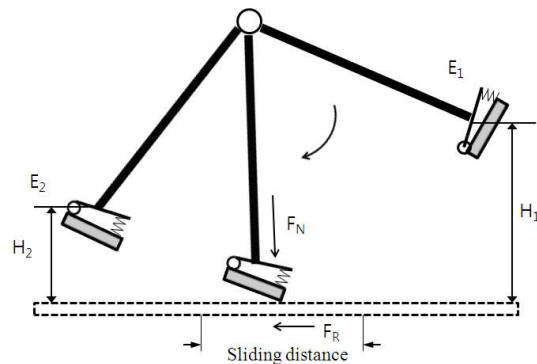
(그림 2) 마찰계수 측정 원리
