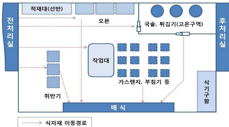
(그림 2) 조리기계·기구 배치(예)
