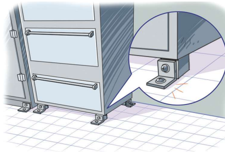
(그림 9) 오븐 기초고정(앵커볼트 취부)
