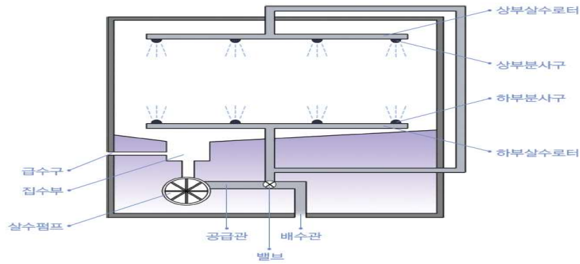
(그림 10) 자동 식기세척기의 구조
