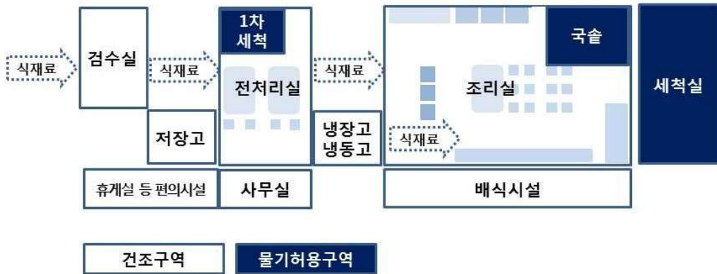
(그림 1) 급식실의 건조구역과 물기허용구역 구분(예)
