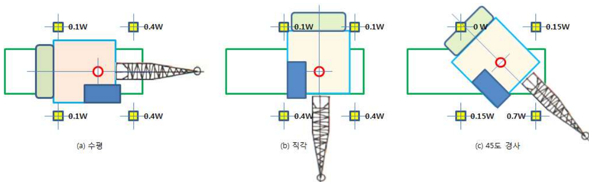
<그림 13> 트럭 크레인 아웃트리거에 대한 하중 배분
