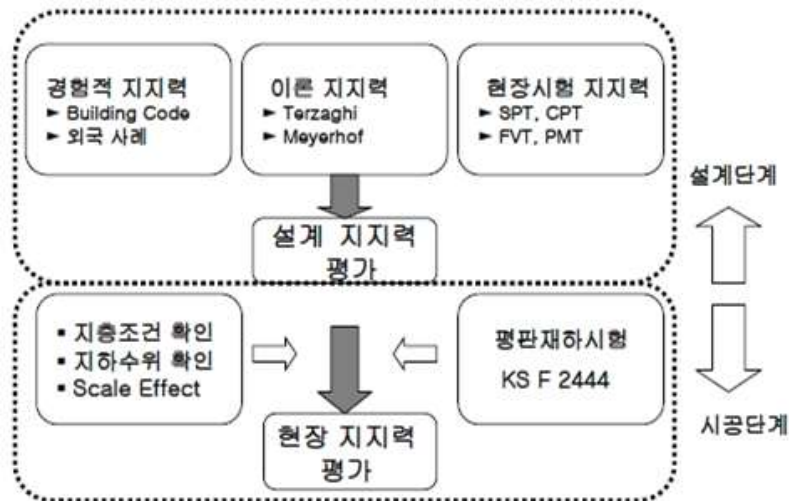
<그림 16> 토사 지지력 평가방법
