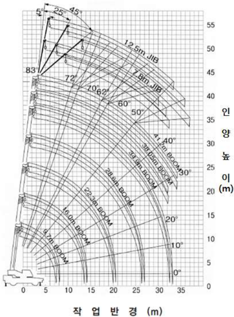
<그림 9> 작업반경과 인양높이 예
