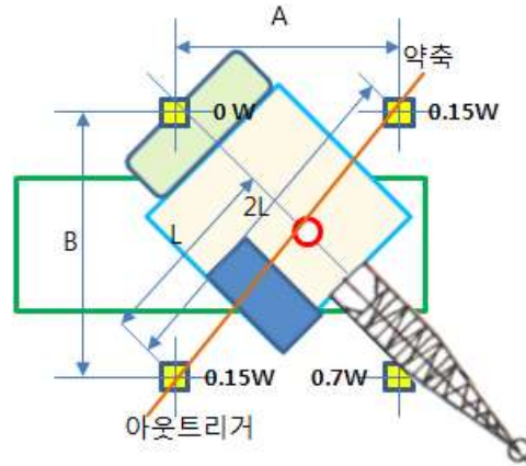
<그림 15> 최대반력계산
