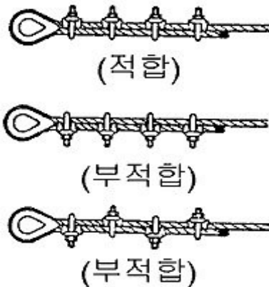
<그림 14> 클립 체결법
