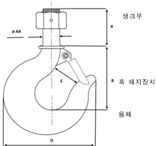
<그림 4> 생크 훅(Shank Hook)
