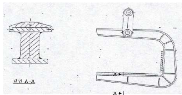
<그림 1> 코일 운반 보조용 달기기구
