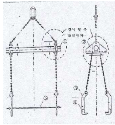
<그림 2> 철판운반 보조용 달기기구
