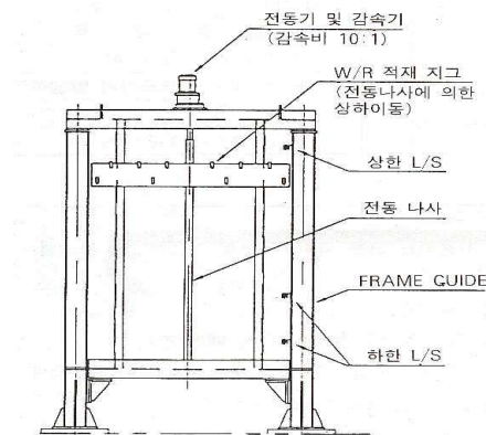
<그림 10> 중형 와이어로프 적치대
