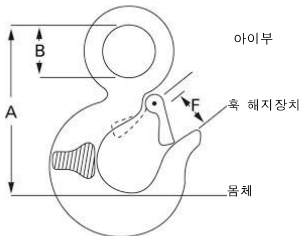
<그림 5> 아이 훅(Eye Hook)
