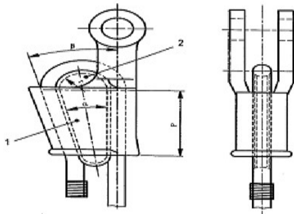
1. 소켓 몸체, 2. 웨지, \alpha . 웨지각, \beta . 소켓각, P. 클램핑 최소길이 <그림 15> 비대칭 웨지소켓
