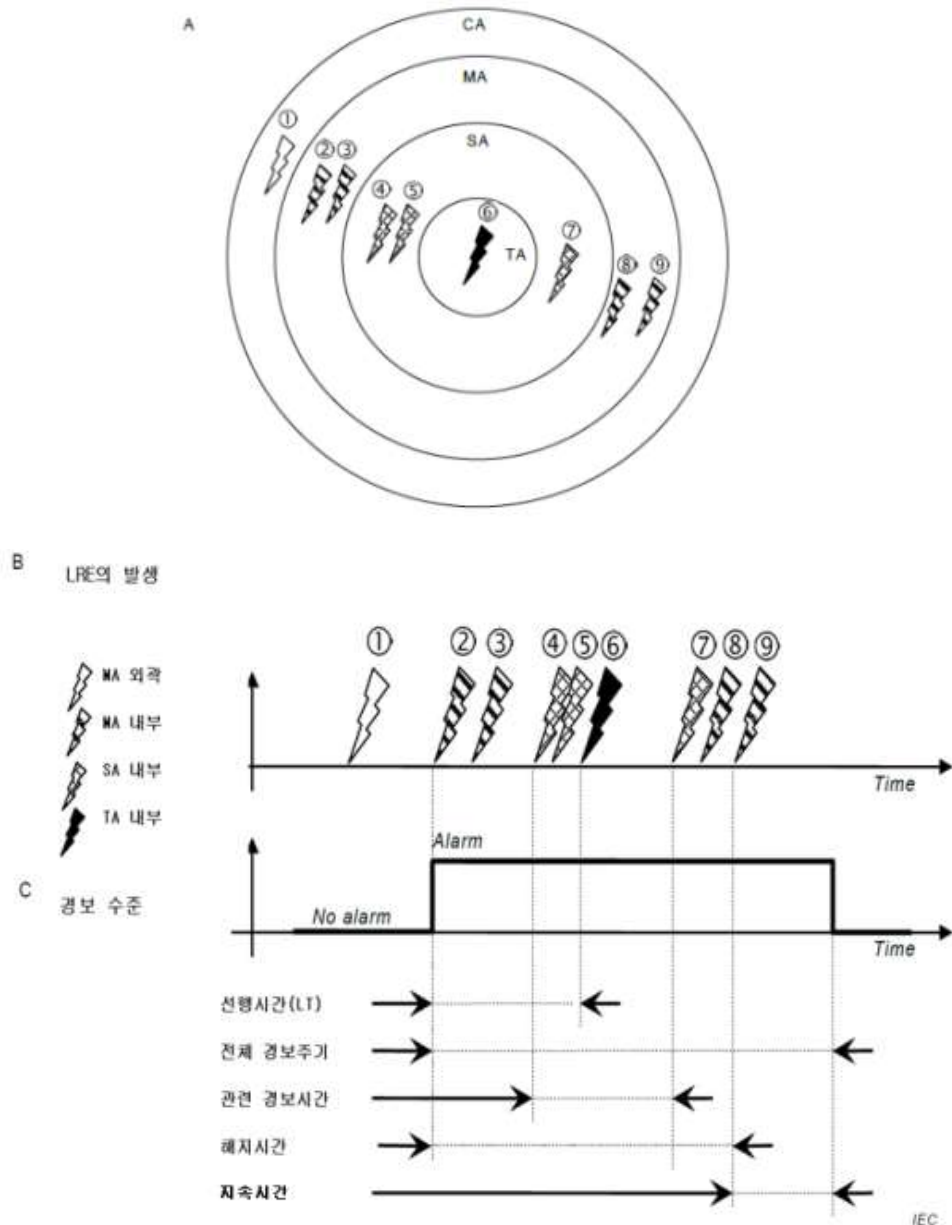
<그림 16> 경보의 예
