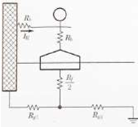
a) 접촉전압 인가 상태
