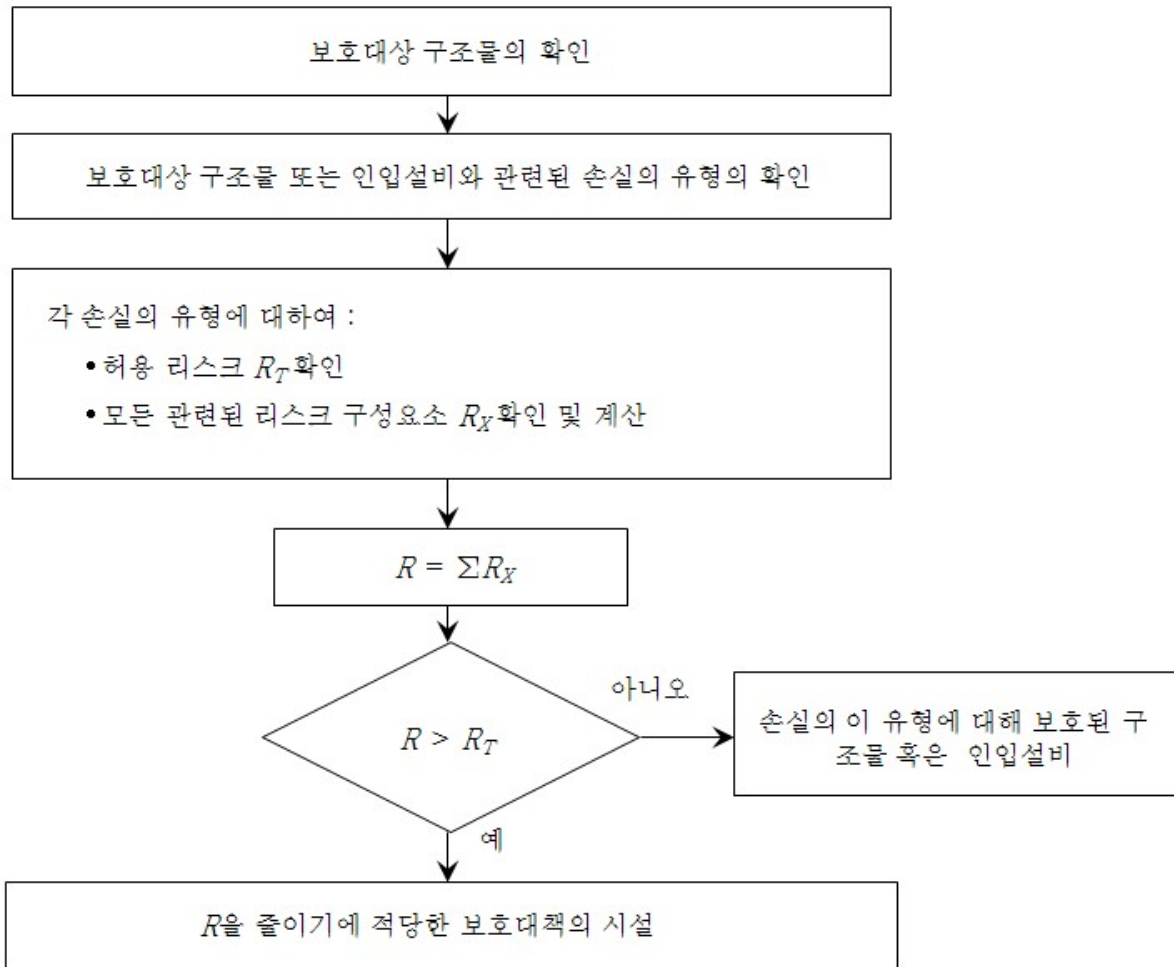
<그림 1> 보호 필요성을 결정하는 절차
