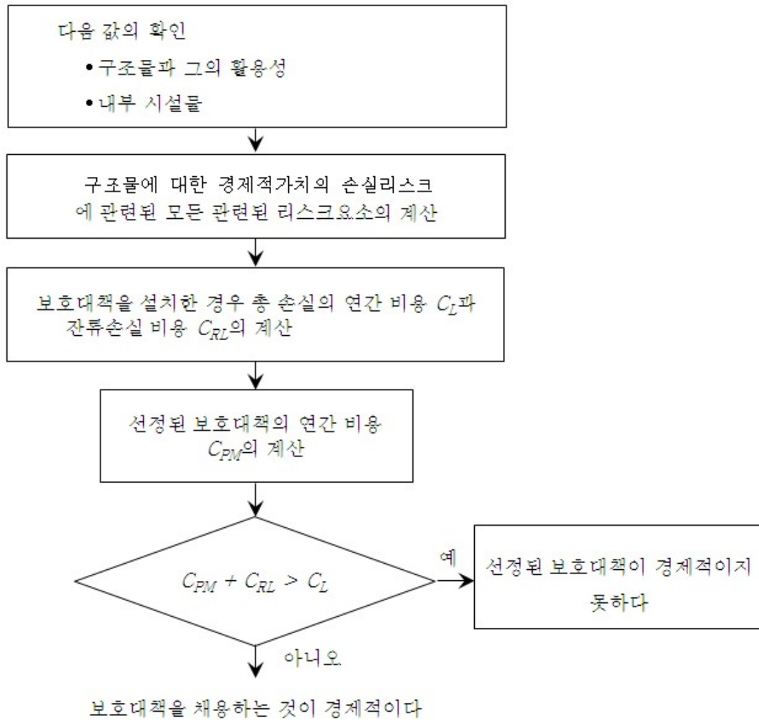
<그림 2> 보호대책의 비용효과를 평가하는 절차
