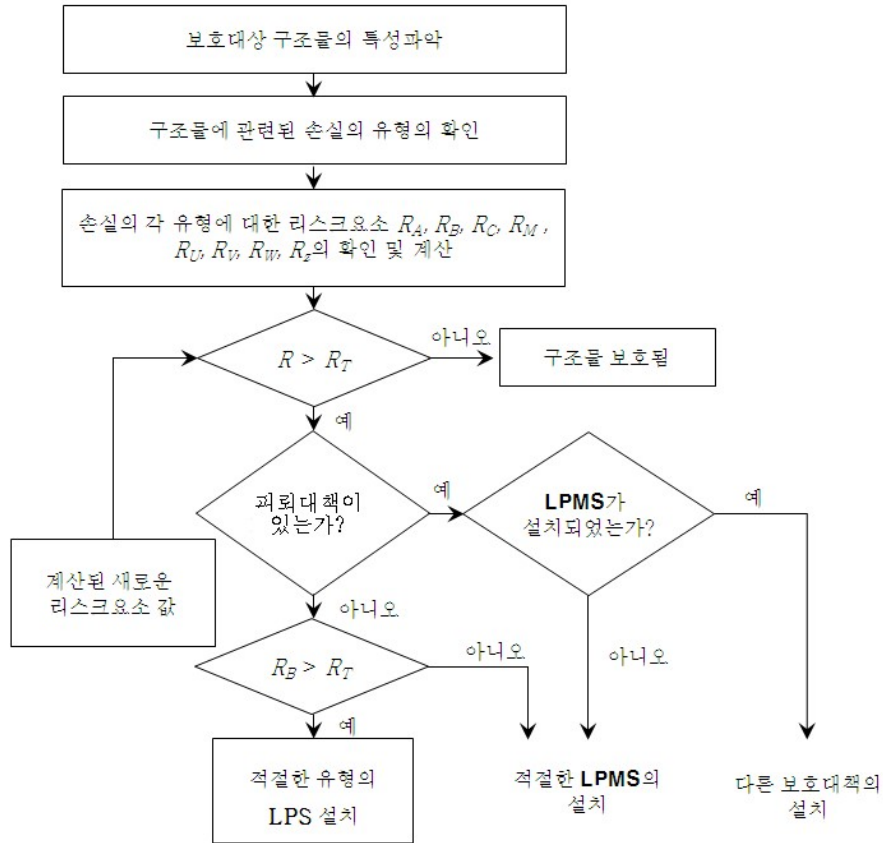
<그림 3> 구조물의 보호대책에 관한 선정절차
