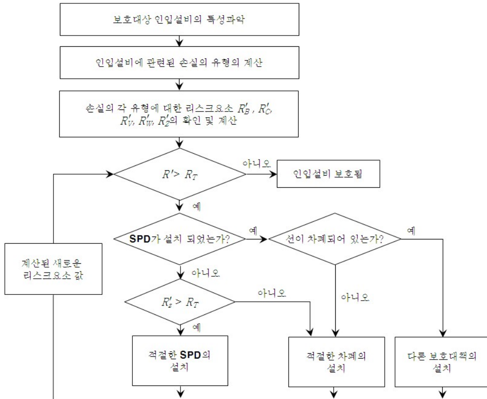
<그림 4> 인입설비의 보호대책에 관한 선정절차
