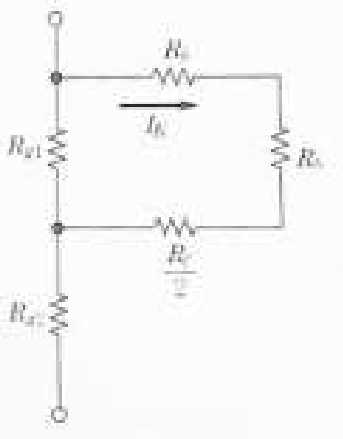
b) 접촉전압 등가회로
