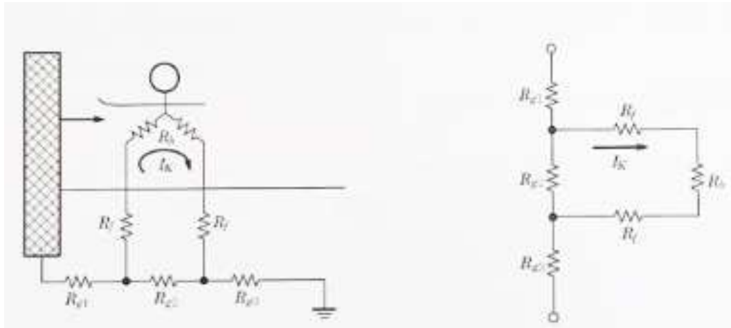
a) 보폭전압 인가 상태
