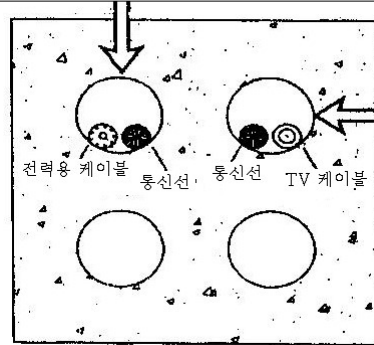
<그림 28> 동일 덕트 내 전력용 케이블 및 약전류 전선
