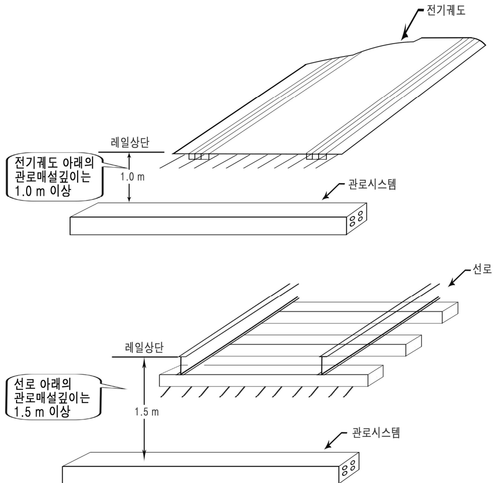
<그림 8> 전기케이블 및 선로와 지하 구조물과의 이격거리
