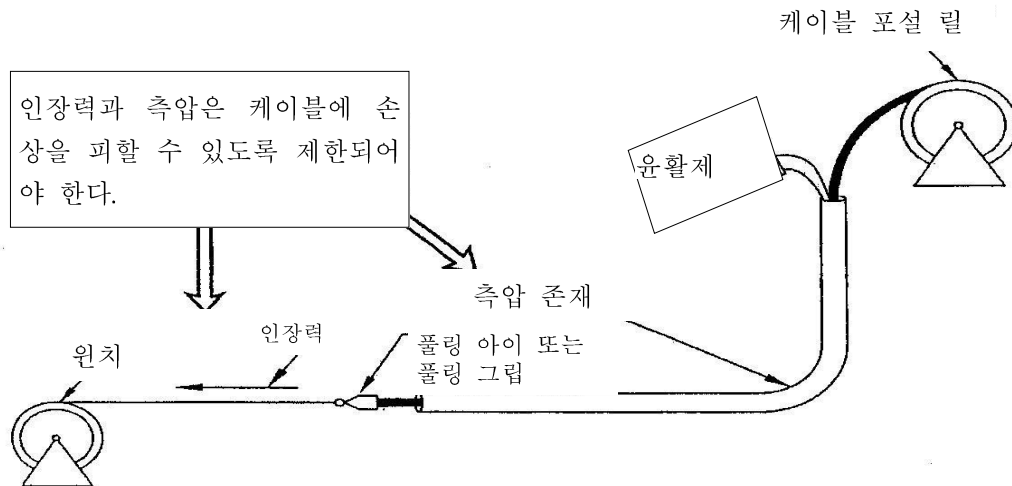
<그림 26> 케이블 인장력과 측압을 줄이는 방법 예
