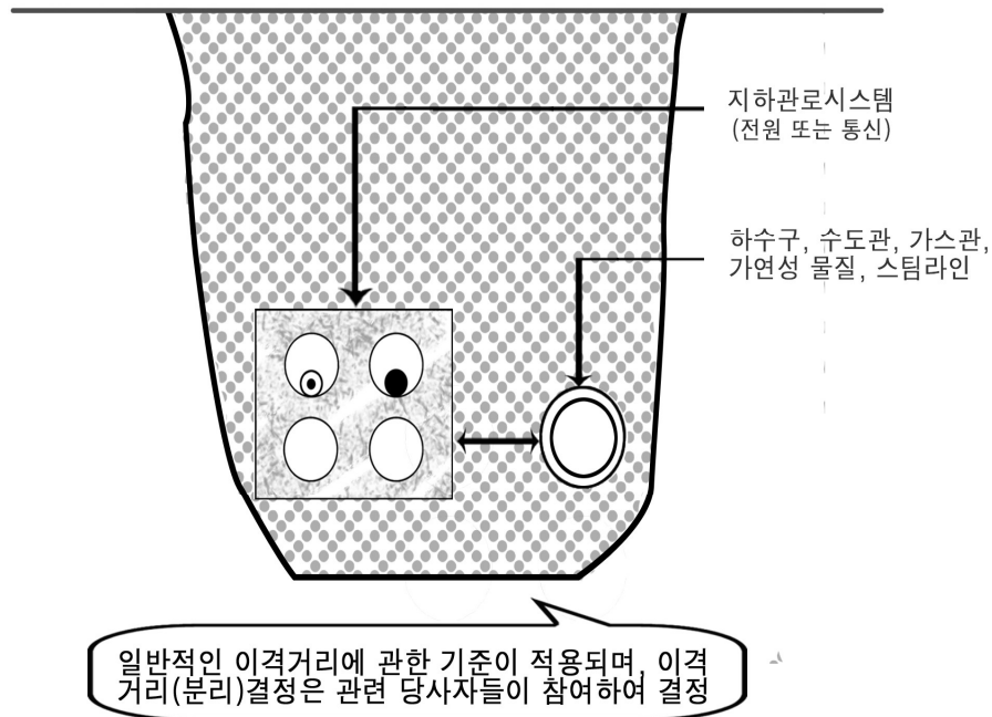
<그림 3> 지중관로와 다른 지하 구조물간의 이격거리
