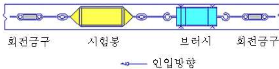
<그림 27> 관로 도통시험 및 청소
