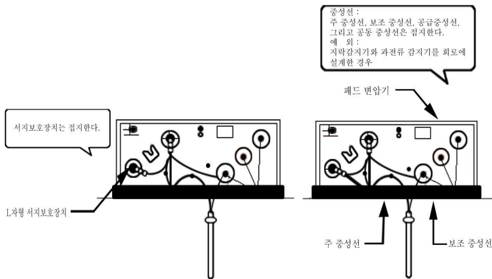
<그림 37> 전선로의 접지
