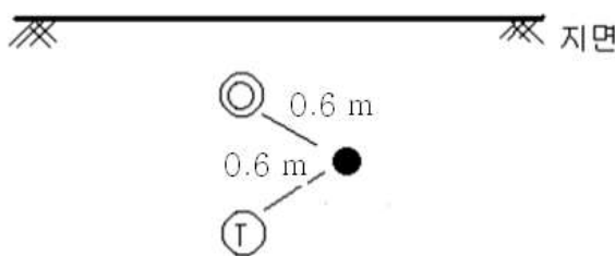
<그림 29> 지중에서 전력용 케이블 및 약전류 전선의 이격거리
