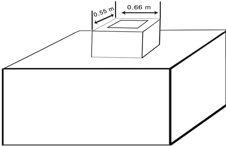
<그림 16> 직사각형 맨홀의 출입구 크기
