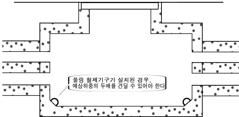
<그림 14> 금속재 롤링의 맨홀 설치 예
