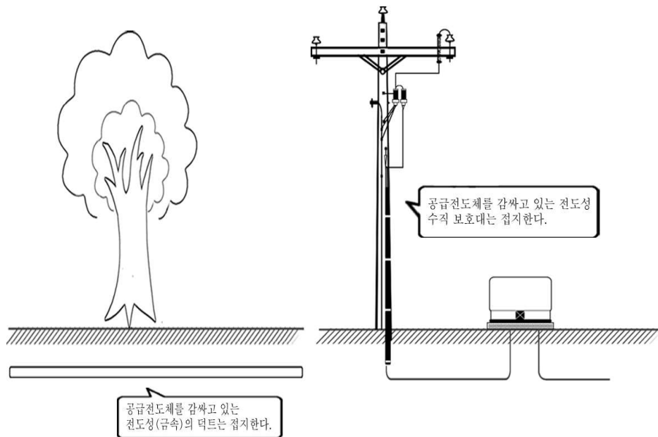
<그림 36> 접지된 도전부
