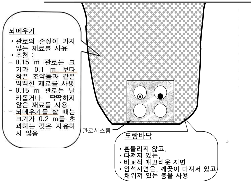
<그림 10> 지중관로의 굴착과 되메우기 방법
