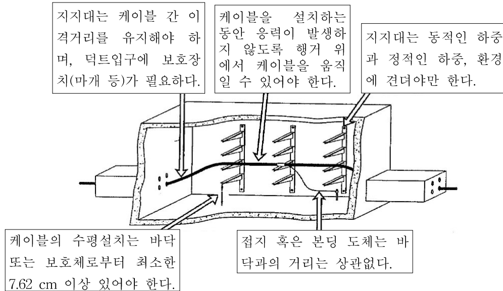
<그림 30> 맨홀 내의 케이블 지지하는 방법
