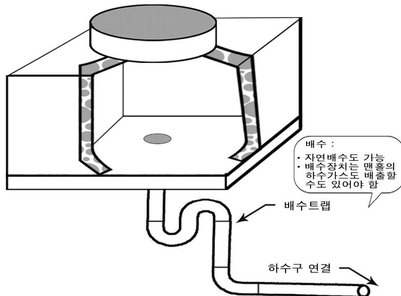
<그림 20> 맨홀내의 배수구 예시
