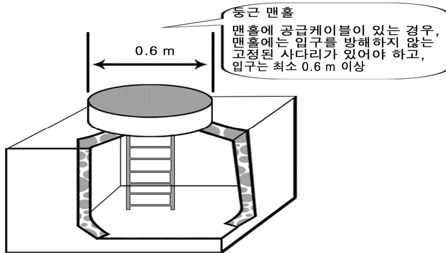
<그림 18> 맨홀내의 사다리 설치 예
