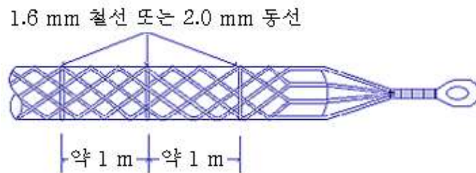
<그림 25> 풀링 그립(pulling grip)
