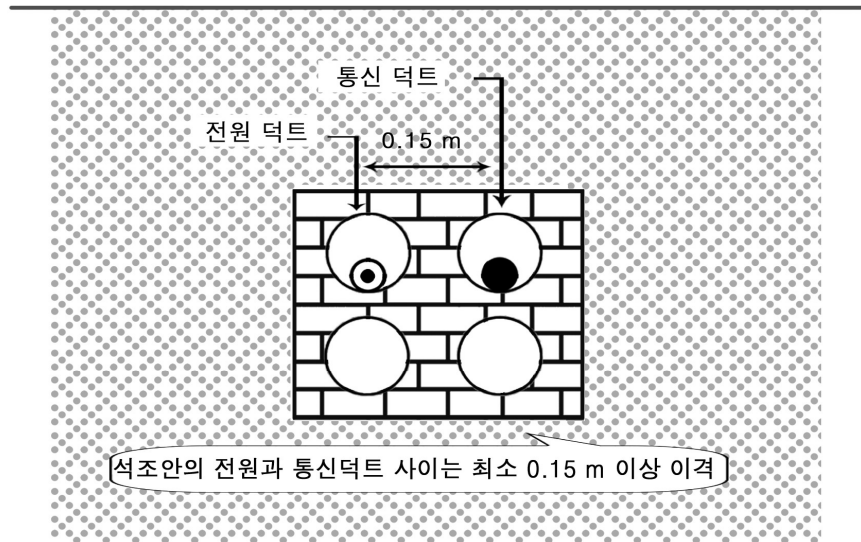
<그림 5> 석조물내에서 전력용과 통신용 덕트의 이격거리
