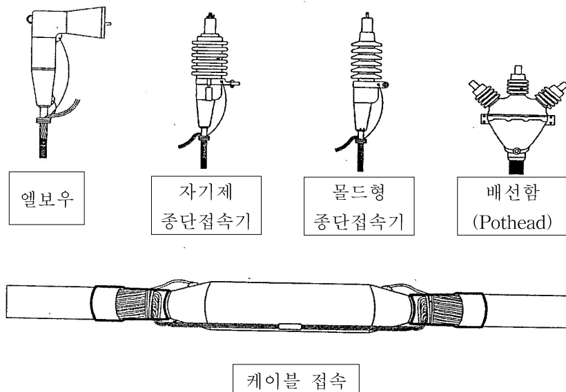
<그림 22> 케이블 접속기구 및 접속의 예
