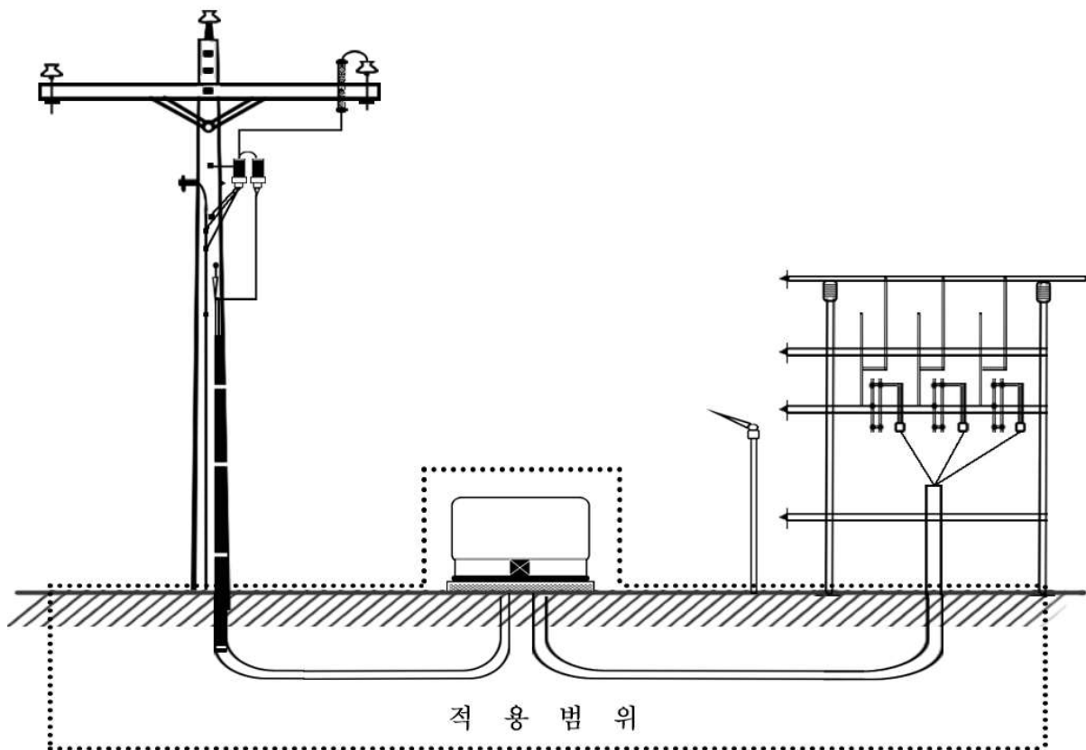
<그림 1>지중선로 등의 적용범위
