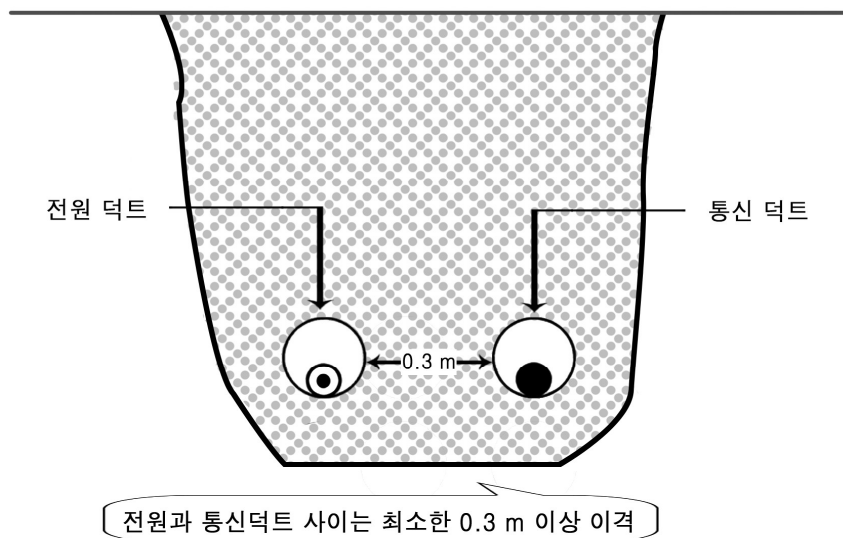
<그림 6> 흙속에서 전력용과 통신용 덕트의 이격거리
