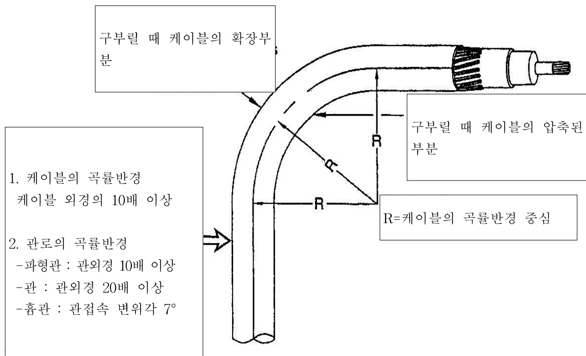
<그림 23> 케이블 곡률반경
