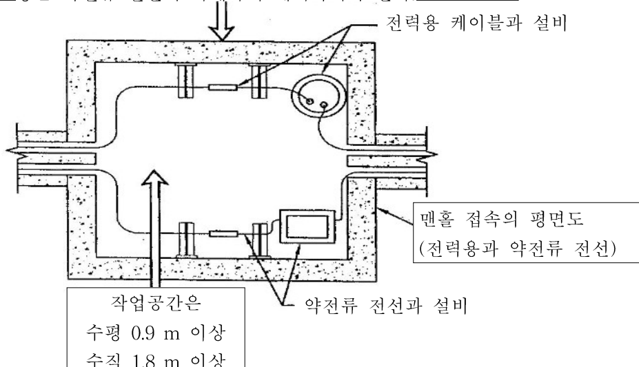
<그림 31> 맨홀 내에서 전력용 및 약전류 전선(장비) 설치방법
