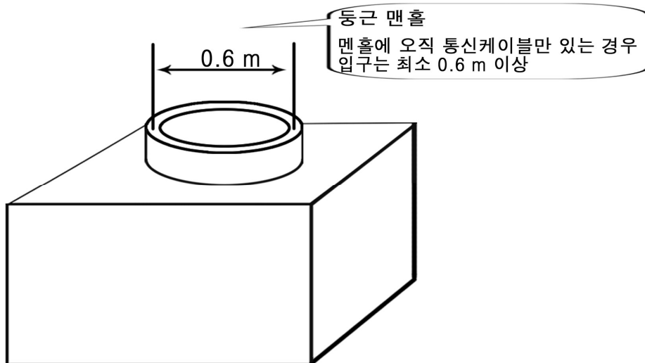
<그림 17> 원형 맨홀의 출입구 크기
