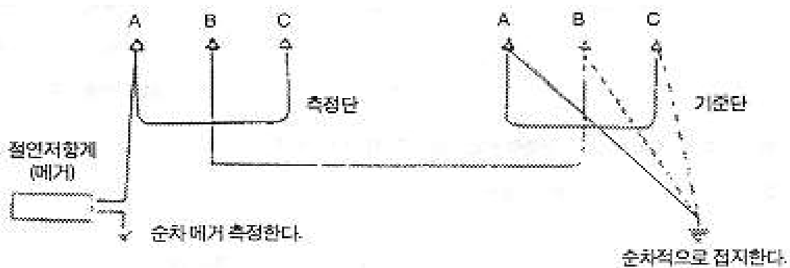
<그림 34> 접지법에 의한 상 확인
