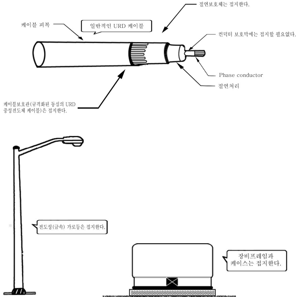
<그림 35> 접지된 도전부
