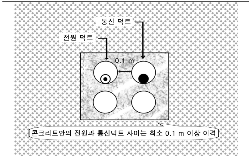
<그림 4> 콘크리트속에서 전력용과 통신용 덕트의 이격거리
