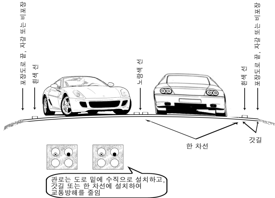
<그림 9> 도로, 고속국도 등의 관로 설치 위치
