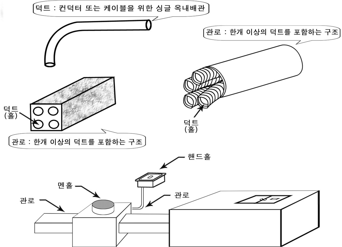
<그림 2> 지중관로 시설의 적용범위
