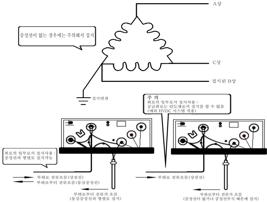
<그림 38> 전선로의 접지
