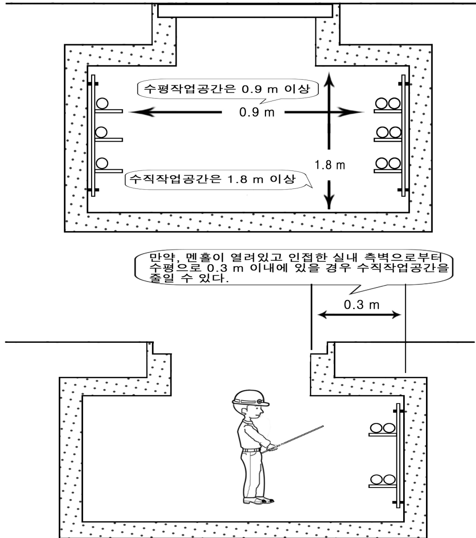
<그림 19> 맨홀내의 작업 공간 크기
