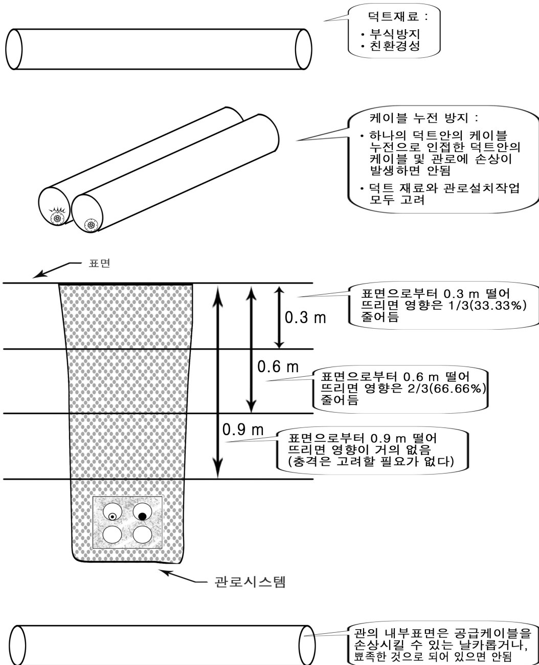
<그림 11> 관로 재료 및 설치방법
