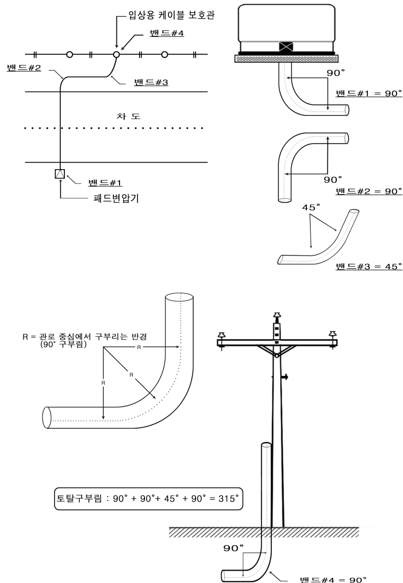
<그림 7> 지중관로의 위치별 곡률반경 예시
