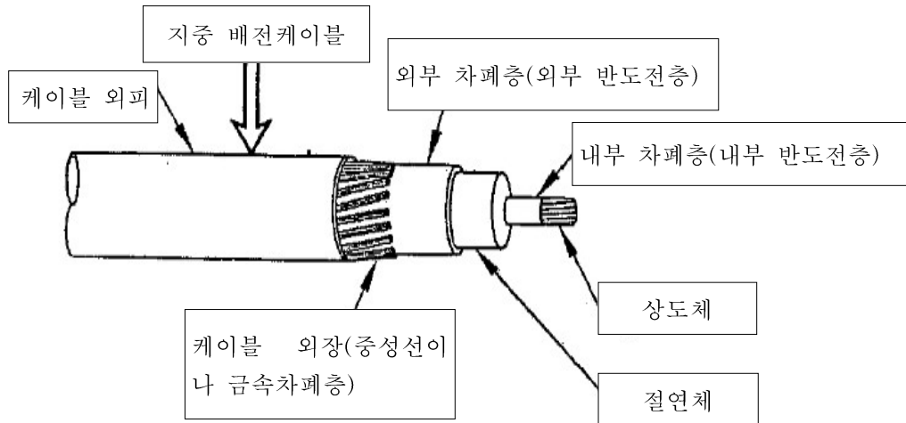
<그림 21> 지중 배전케이블의 외장, 외피 및 차폐층 형식의 예
