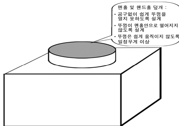
<그림 15> 맨홀 덮개의 설치 모양
